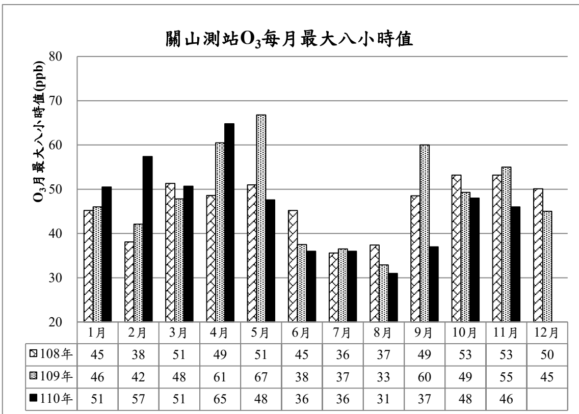
圖 16、近三年 O 3 每月最大八小時值
