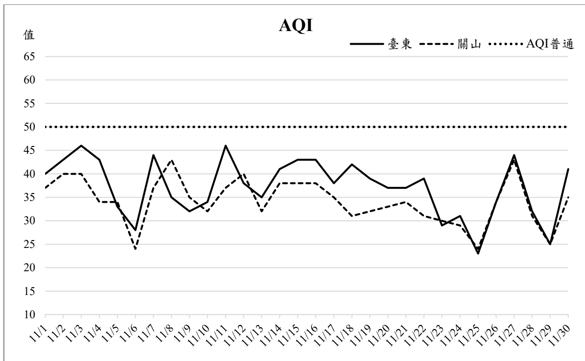
圖 3、110 年 11 月臺東及關山測站空氣品質指標 (AQI) 變化趨勢
