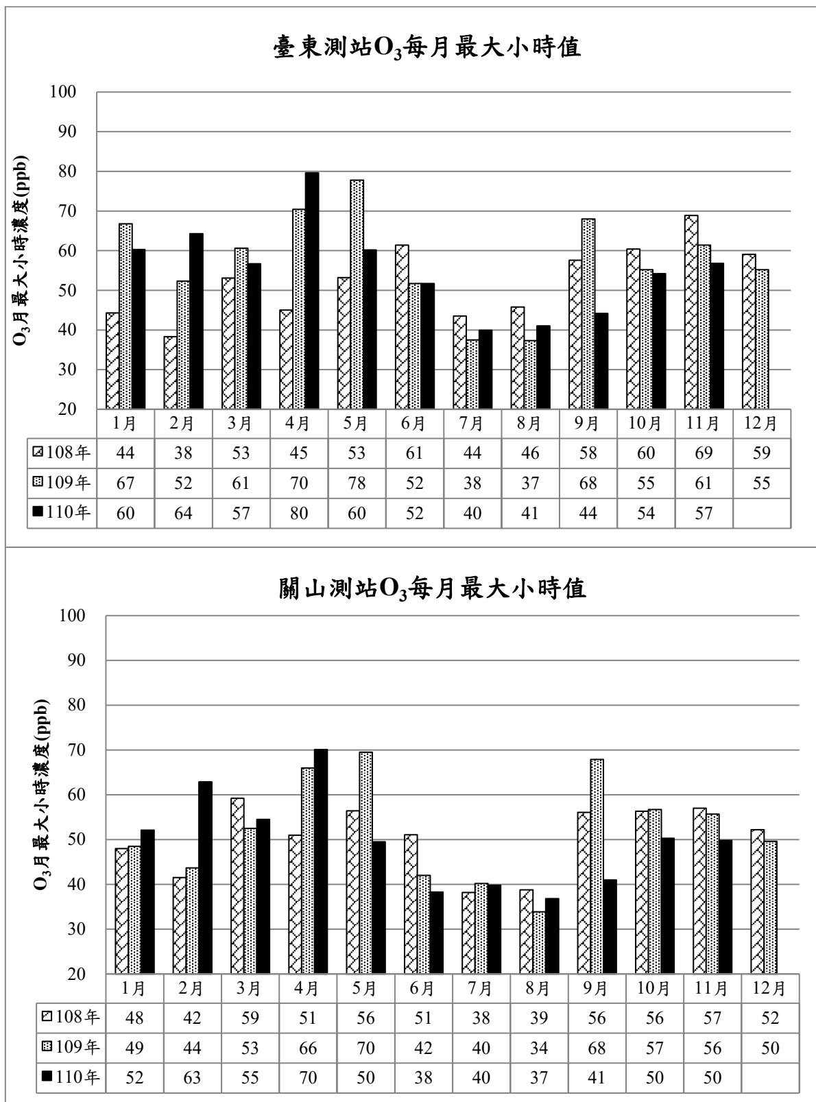
圖 15、近三年 O 3 每月最大小時值
