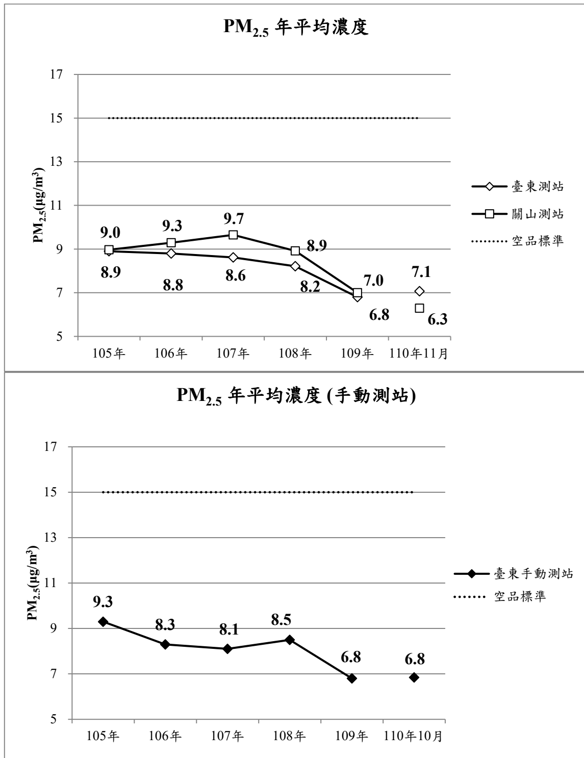
圖 20、臺東環保署測站 PM 2.5 年平均濃度變化
