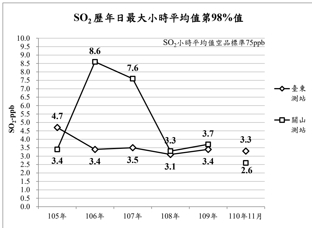
圖 17、SO 2 歷年日最大小時平均值第 98% 值
