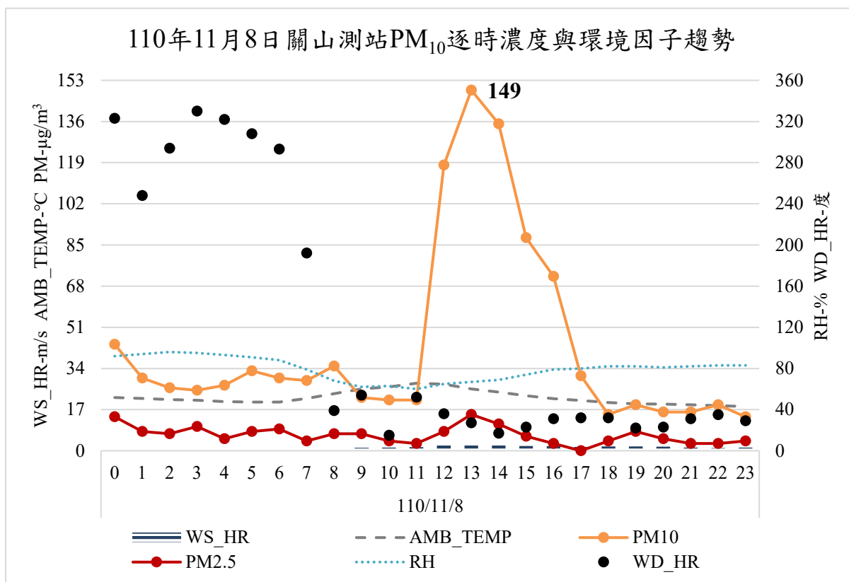
圖 11、110年11月8日關山測站 PM 10 逐時濃度與環境因子趨勢
