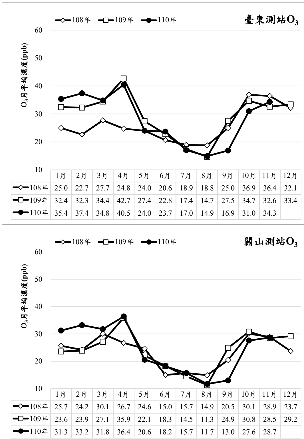
圖 14、近三年臺東及關山測站 O 3 濃度逐月變化趨勢
