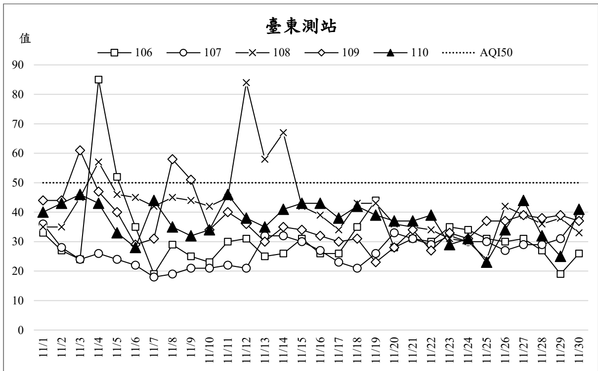
圖 1、近五年 11 月份同期之臺東測站空氣品質指標 (AQI) 變化趨勢
