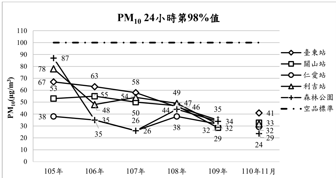
圖 7、臺東縣各測站 PM 10 24 小時第八大值濃度變化
