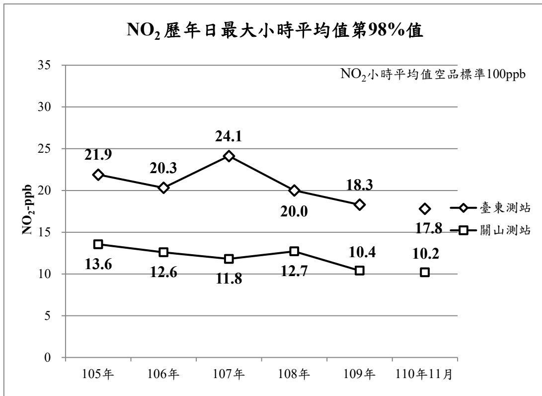
圖 18、NO 2 歷年日最大小時平均值第 98% 值
