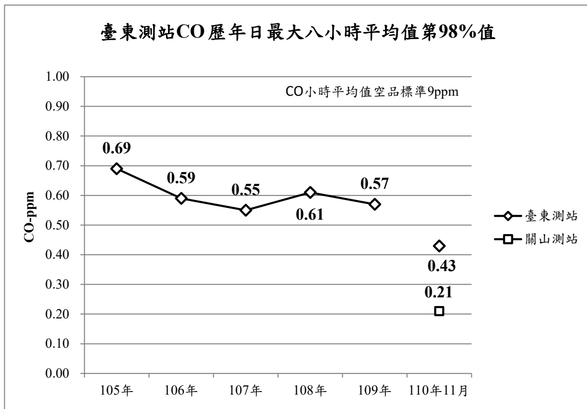
圖 19、臺東測站 CO 歷年日最大八小時平均值第 98% 值
