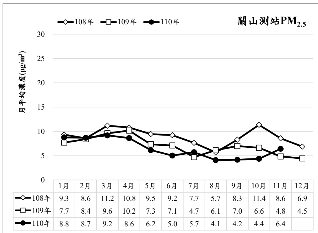
圖 22、近三年 PM 2.5 濃度逐月變化趨勢
