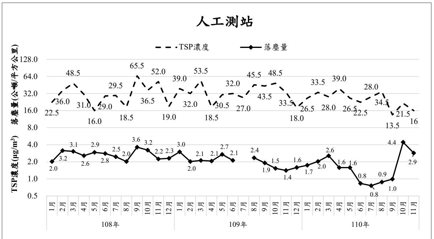
圖 23、臺東環保局人工測站 TSP 與落塵量
