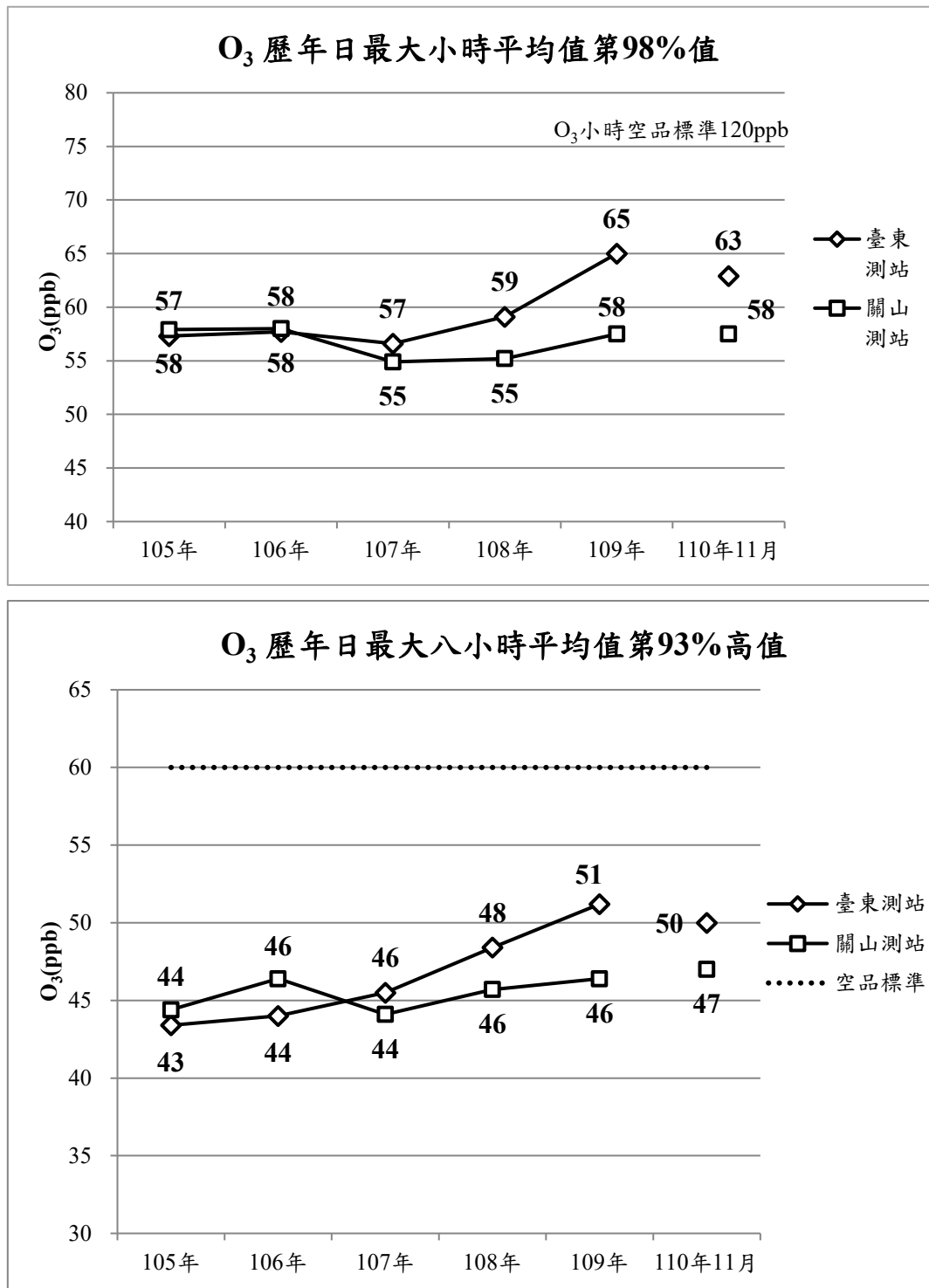
圖 13、臺東環保署測站 O 3 達標程度變化
