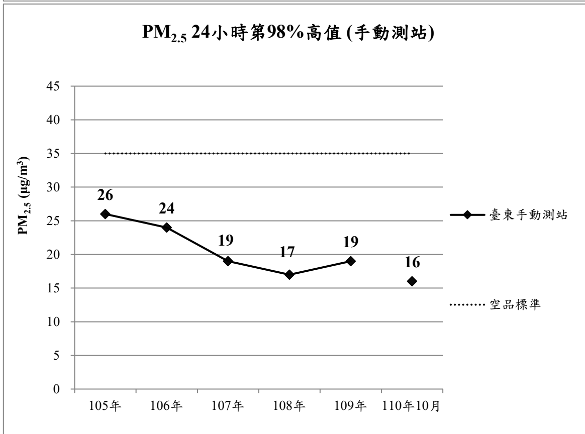
圖 21、臺東環保署測站 PM 2.5 達標程度變化
