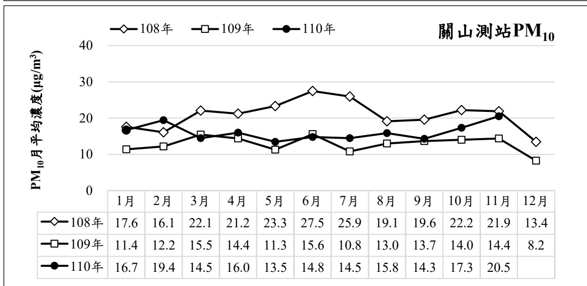
圖 8、近三年臺東及關山測站 PM 10 濃度逐月變化趨勢
