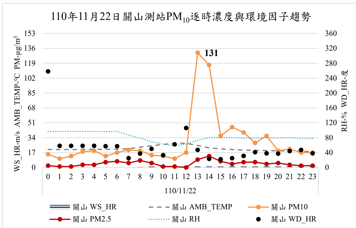
圖 12、110年11月22日關山測站 PM 10 逐時濃度與環境因子趨勢
