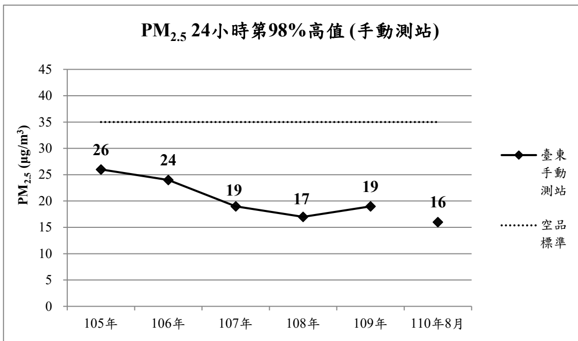
圖 19、臺東環保署測站 PM 2.5 達標程度變化
