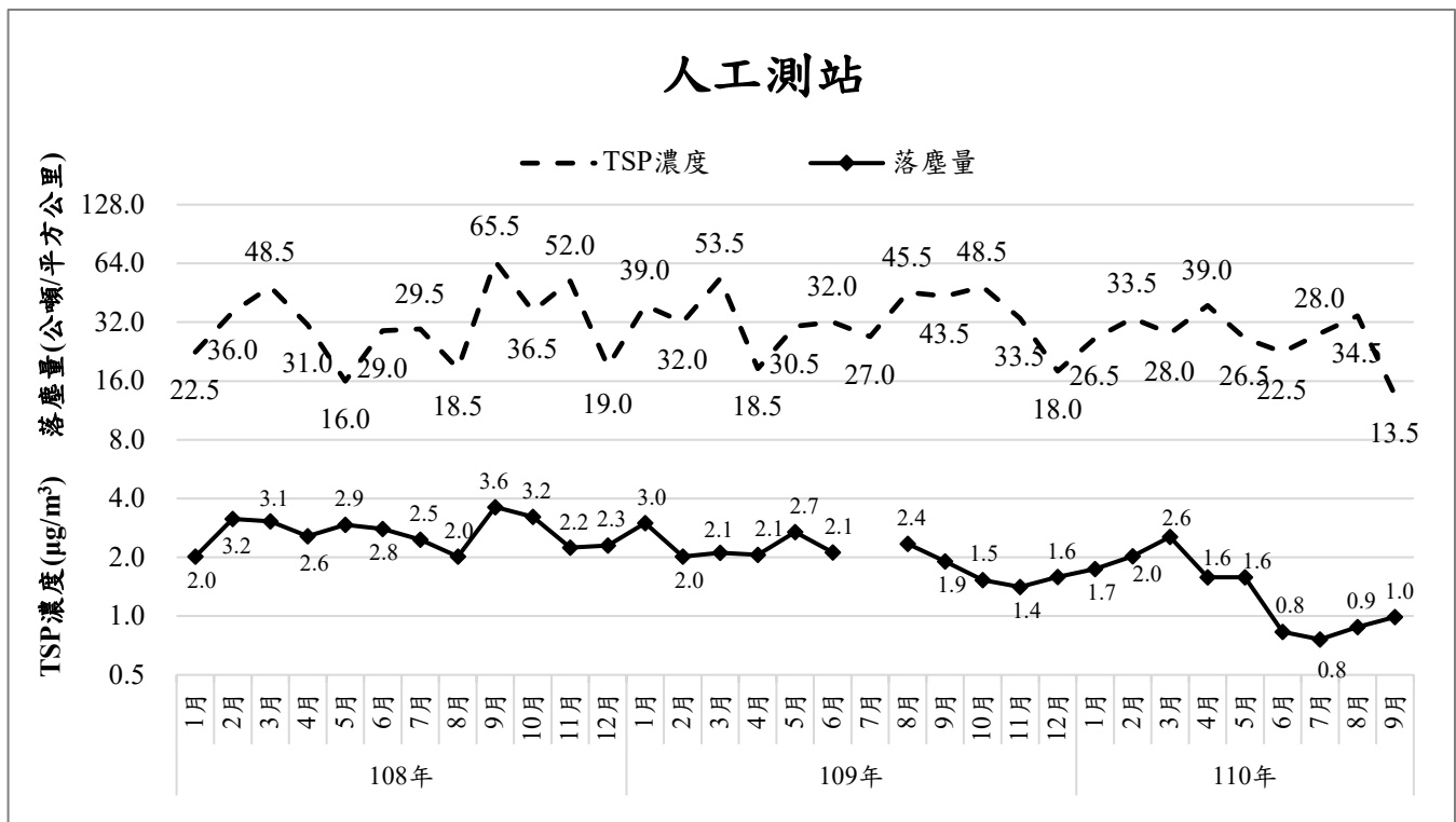
圖 21、臺東環保局人工測站 TSP 與落塵量
