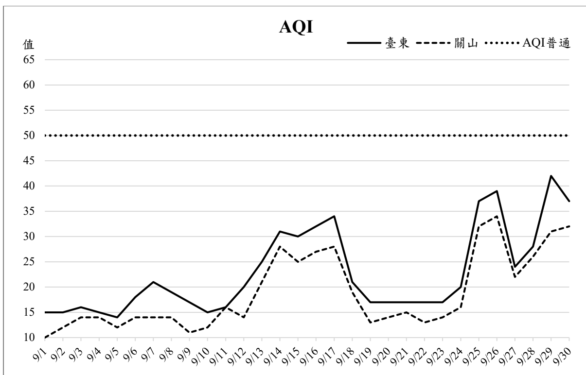
圖 3、110年9月臺東及關山測站空氣品質指標(AQI)變化趨勢
