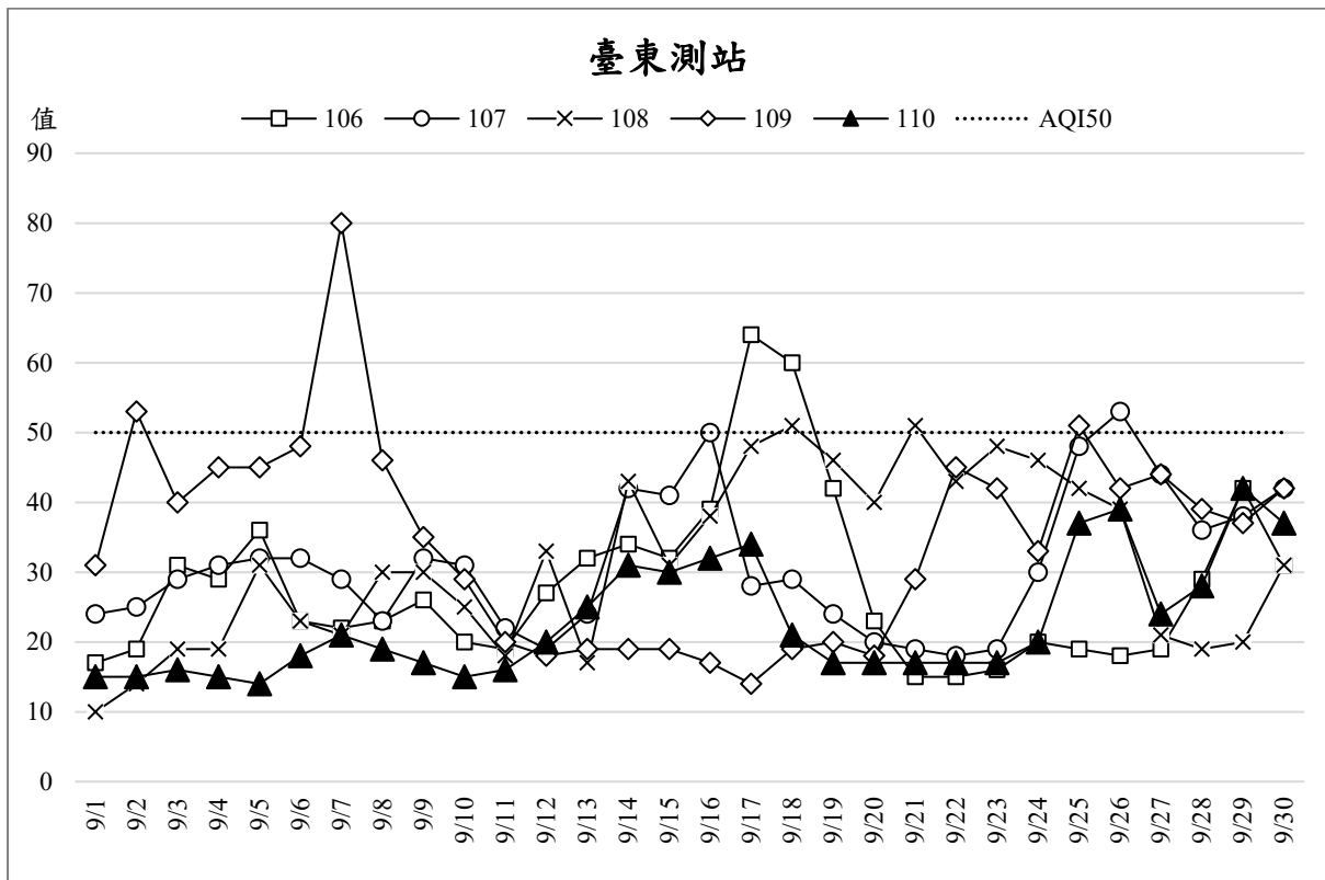
圖 1、近五年 9 月份同期之臺東測站空氣品質指標 (AQI) 變化趨勢
