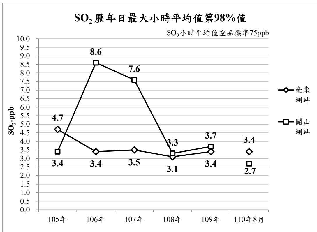
圖 15、SO 2 歷年日最大小時平均值第 98% 值
