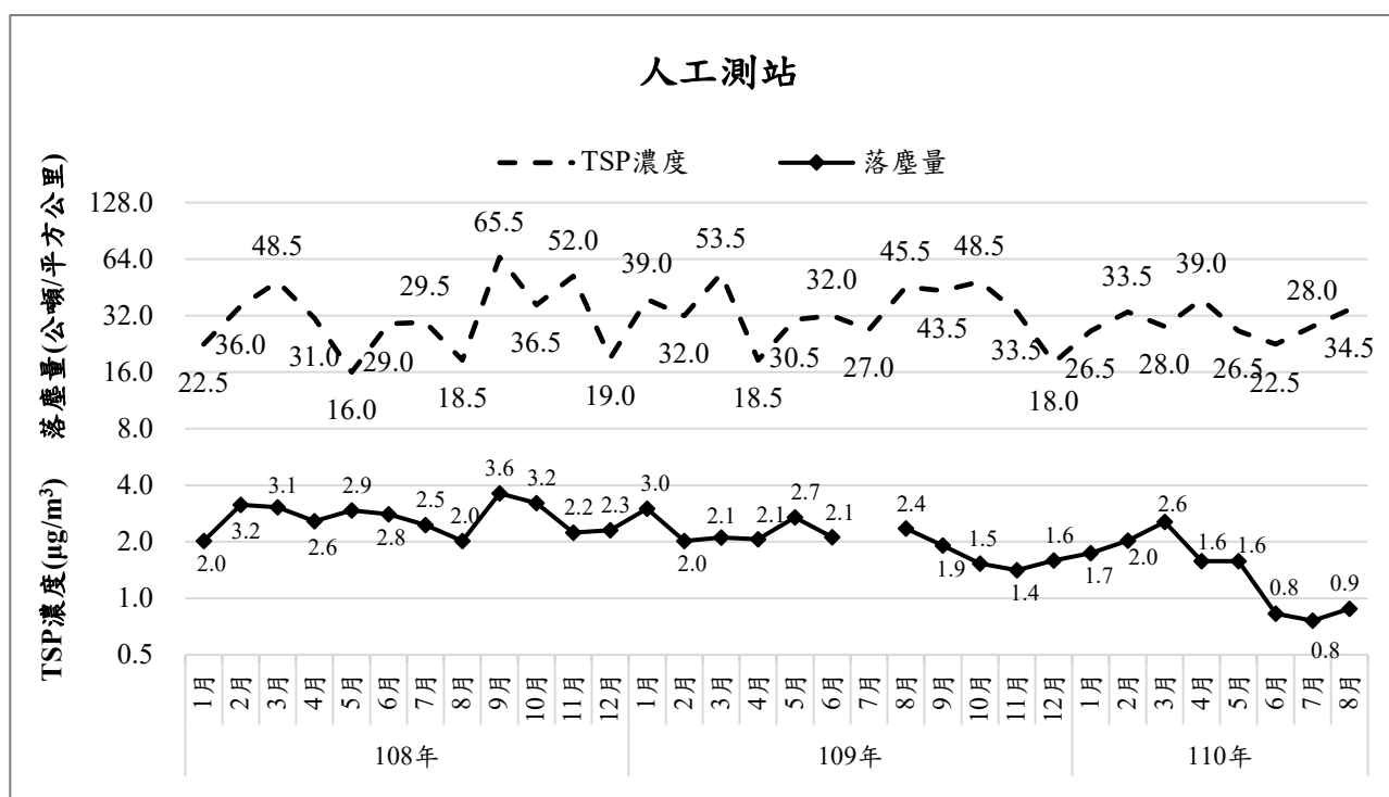
圖 21、臺東環保局人工測站 TSP 與落塵量
