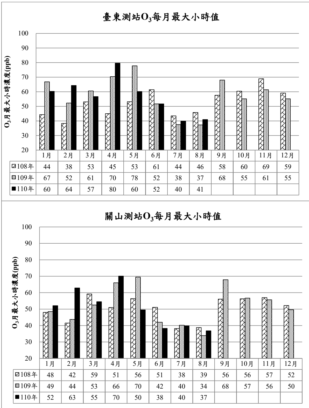
圖 13、近三年 O 3 每月最大小時值
