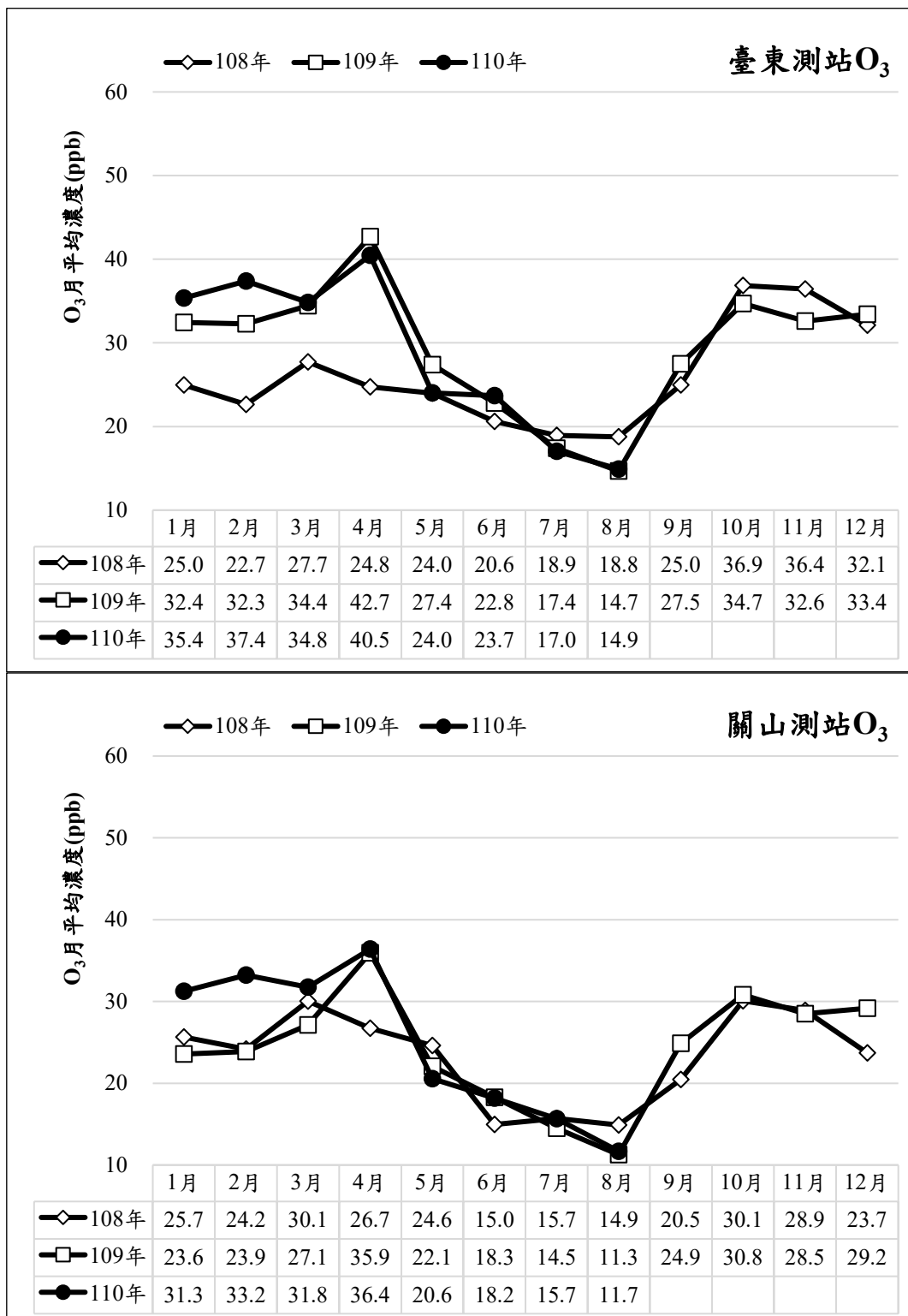
圖 12、近三年臺東及關山測站 O 3 濃度逐月變化趨勢
