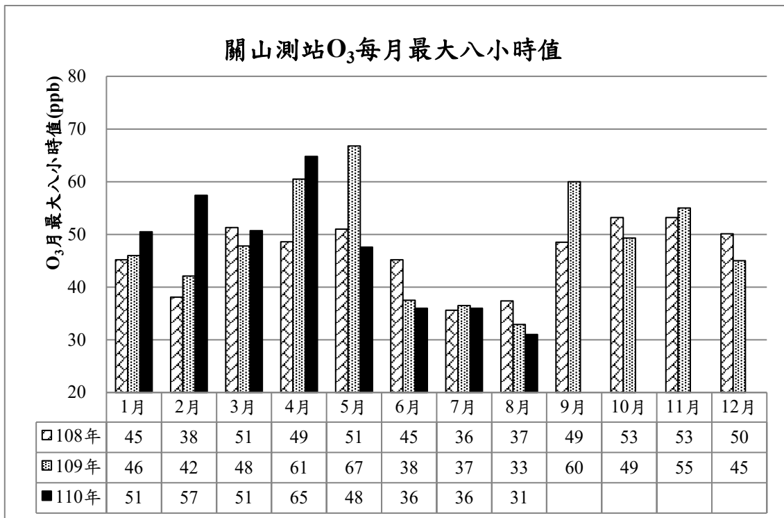
圖 14、近三年 O 3 每月最大八小時值
