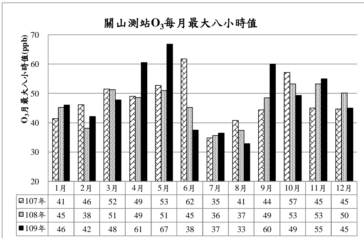
圖 14、近三年 O 3 每月最大八小時值
