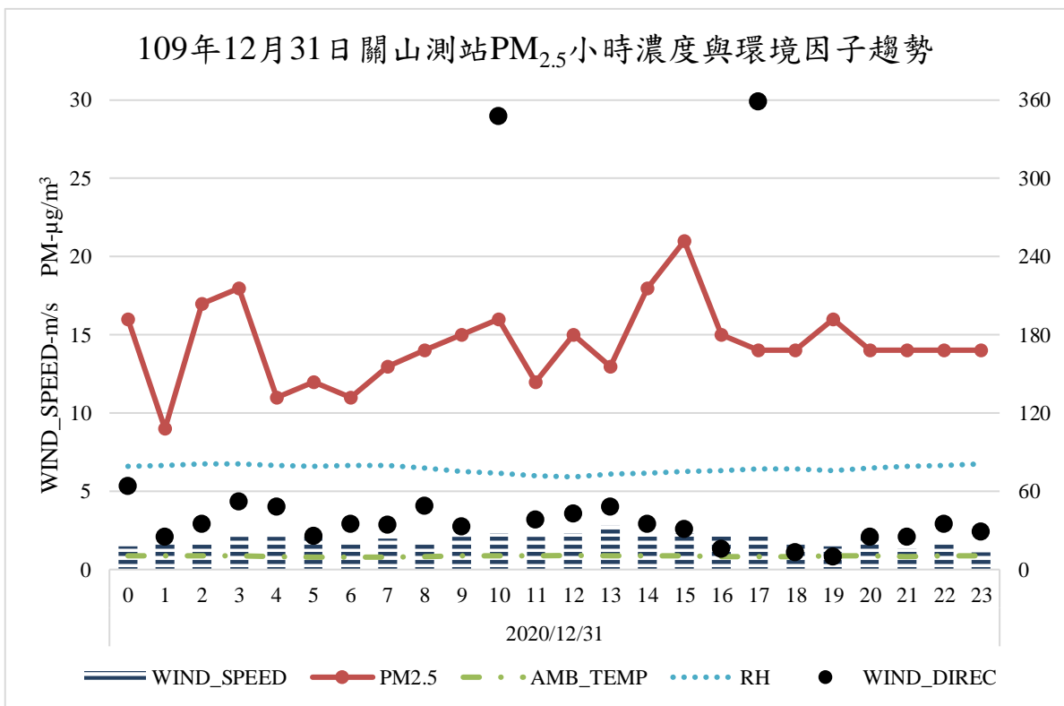
圖 22、109 年 12 月 31 日關山測站 PM 2.5 小時濃度與環境因子趨勢
