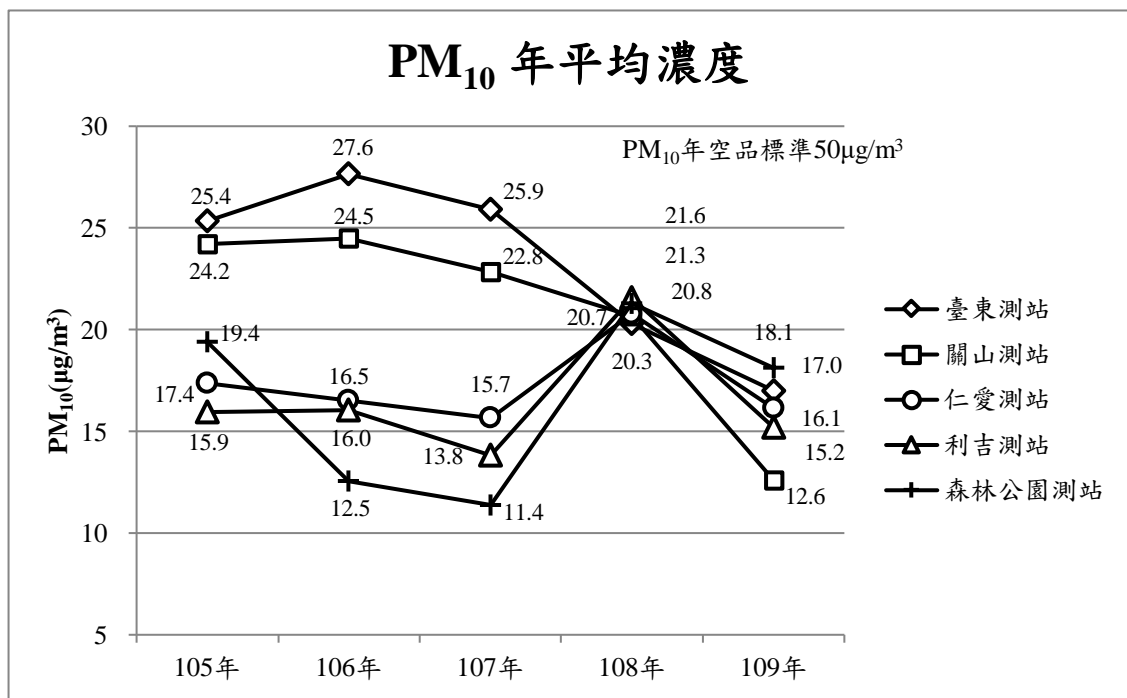
圖 6、臺東縣各測站 \text{PM}_{10} 年平均濃度變化
