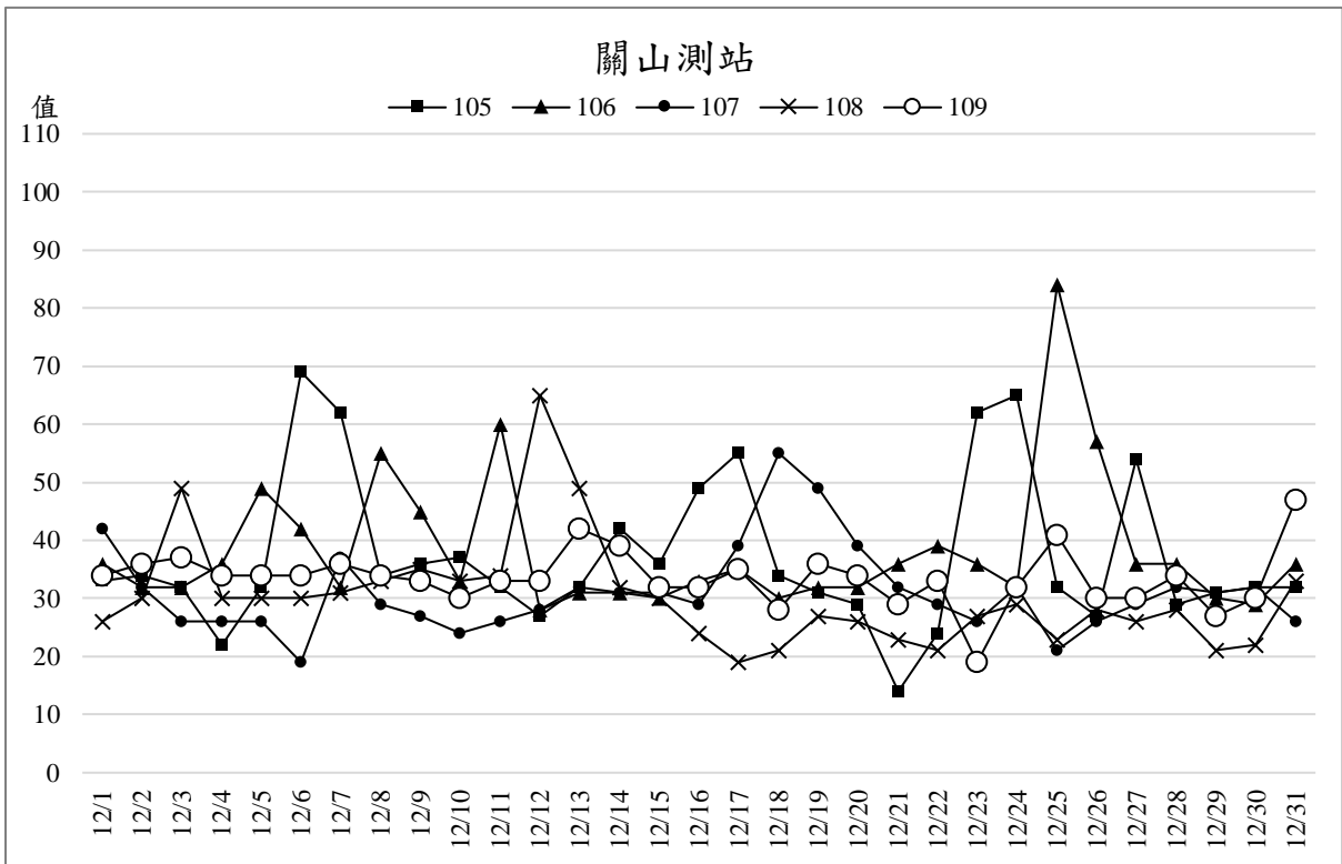
圖 2、近五年 12 月份同期之關山測站空氣品質指標 (AQI) 變化趨勢
