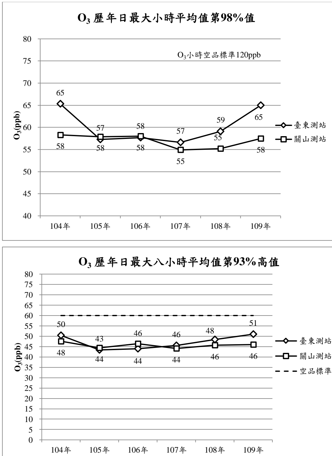
圖 11、臺東環保署測站 O 3 達標程度變化
