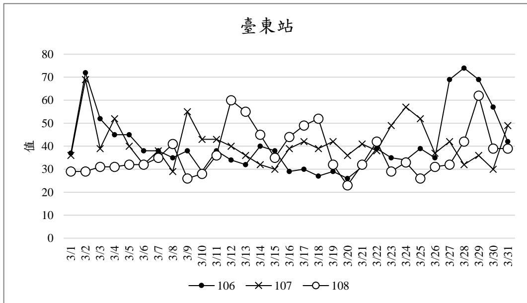
圖 1 近三年 3 月份同期之臺東站空氣品質指標 (AQI) 變化趨勢
