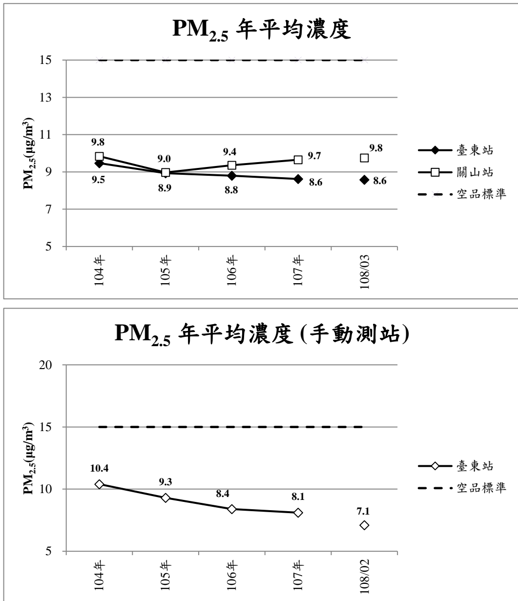
圖 17 臺東環保署測站 PM 2.5 年平均濃度變化
