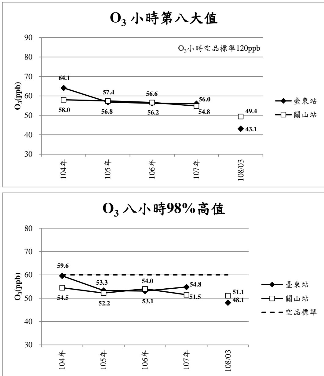
圖 10 臺東環保署測站 O 3 達標程度變化
