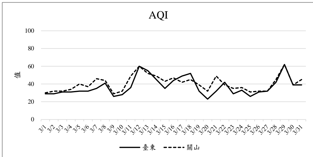
圖 3 108年3月臺東及關山測站空氣品質指標 (AQI) 變化趨勢
