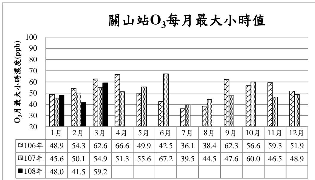
圖 12 近三年 O 3 濃度月最大小時值變化趨勢
