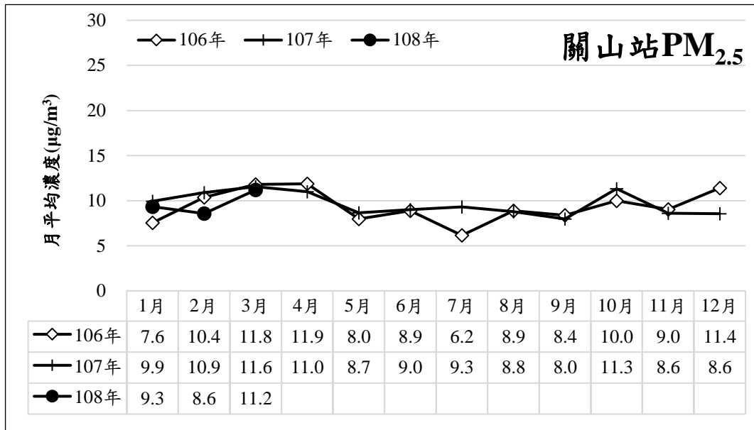
圖 19 近三年 PM 2.5 濃度逐月變化趨勢
