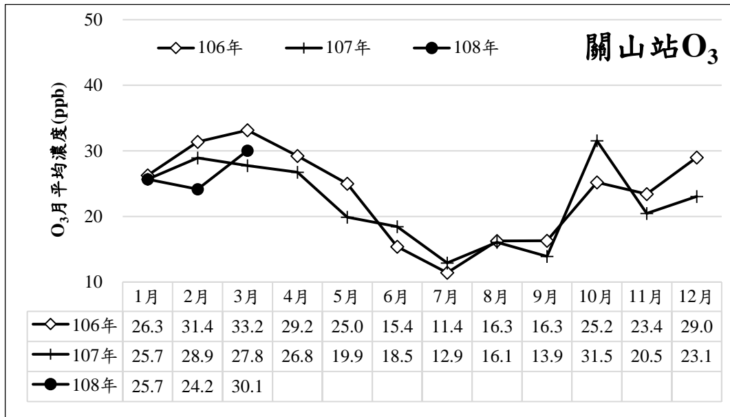
圖 11 近三年 O 3 濃度逐月變化趨勢
