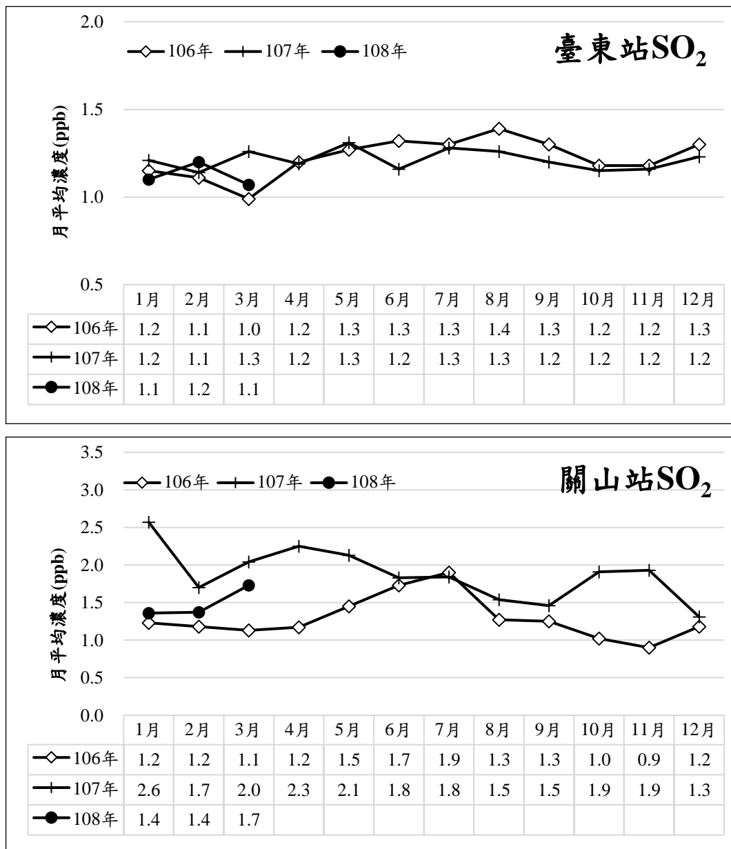
圖 14 近三年 SO 2 濃度逐月變化趨勢
