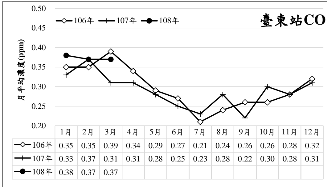
圖 16 近三年 CO 濃度逐月變化趨勢
