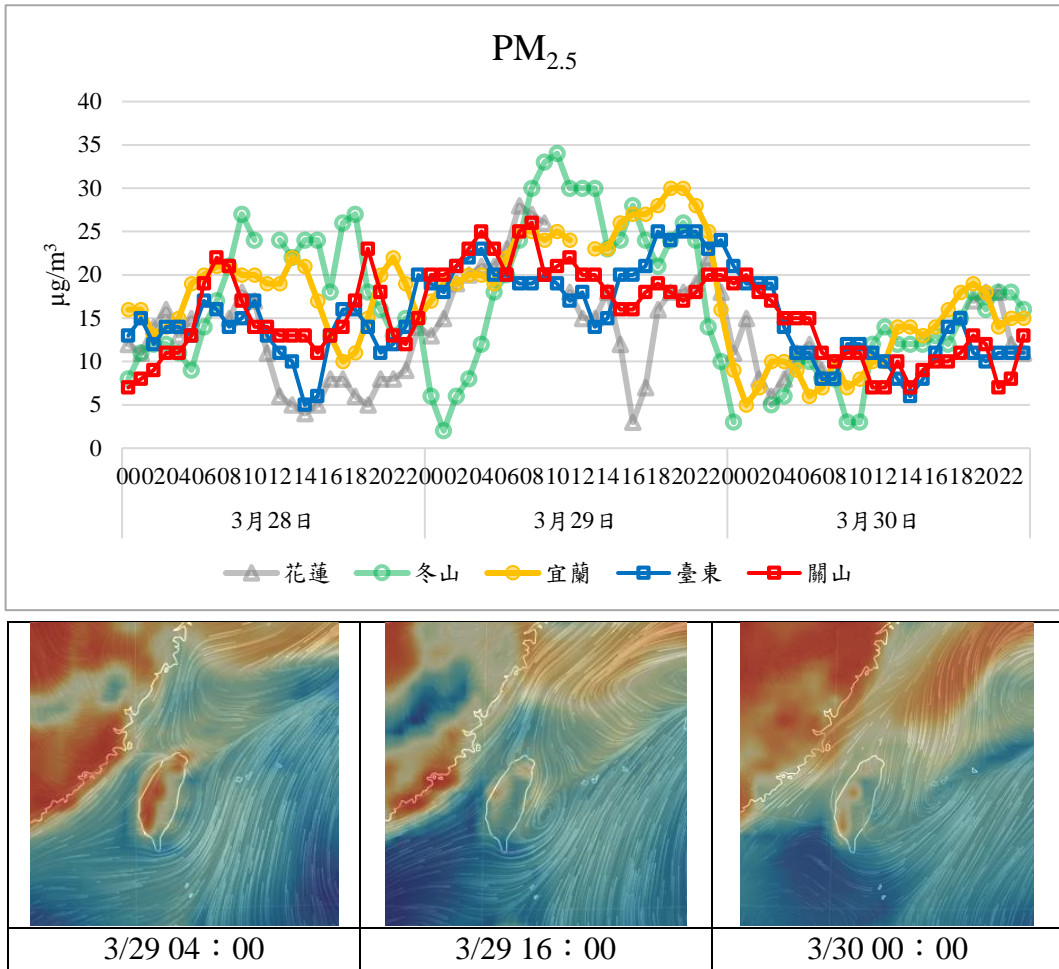
圖 21 3 月 28~30 日東部測站受境外移入影響及風場變化情形
