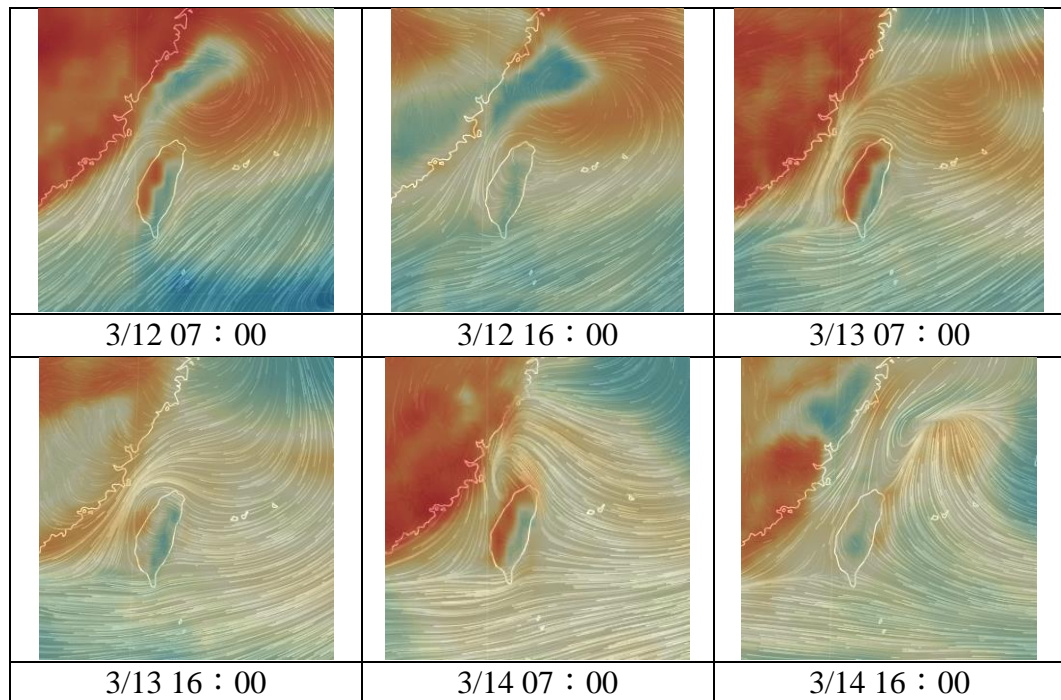
圖 20 3月12~15日東部測站受境外移入影響及風場變化情形
