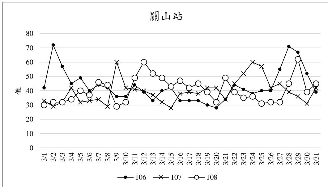
圖 2 近三年 3 月份同期之關山站空氣品質指標 (AQI) 變化趨勢
