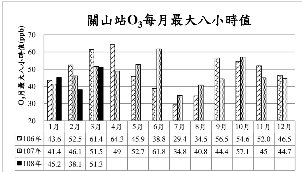
圖 13 近三年 O 3 濃度月最大八小時值變化趨勢
