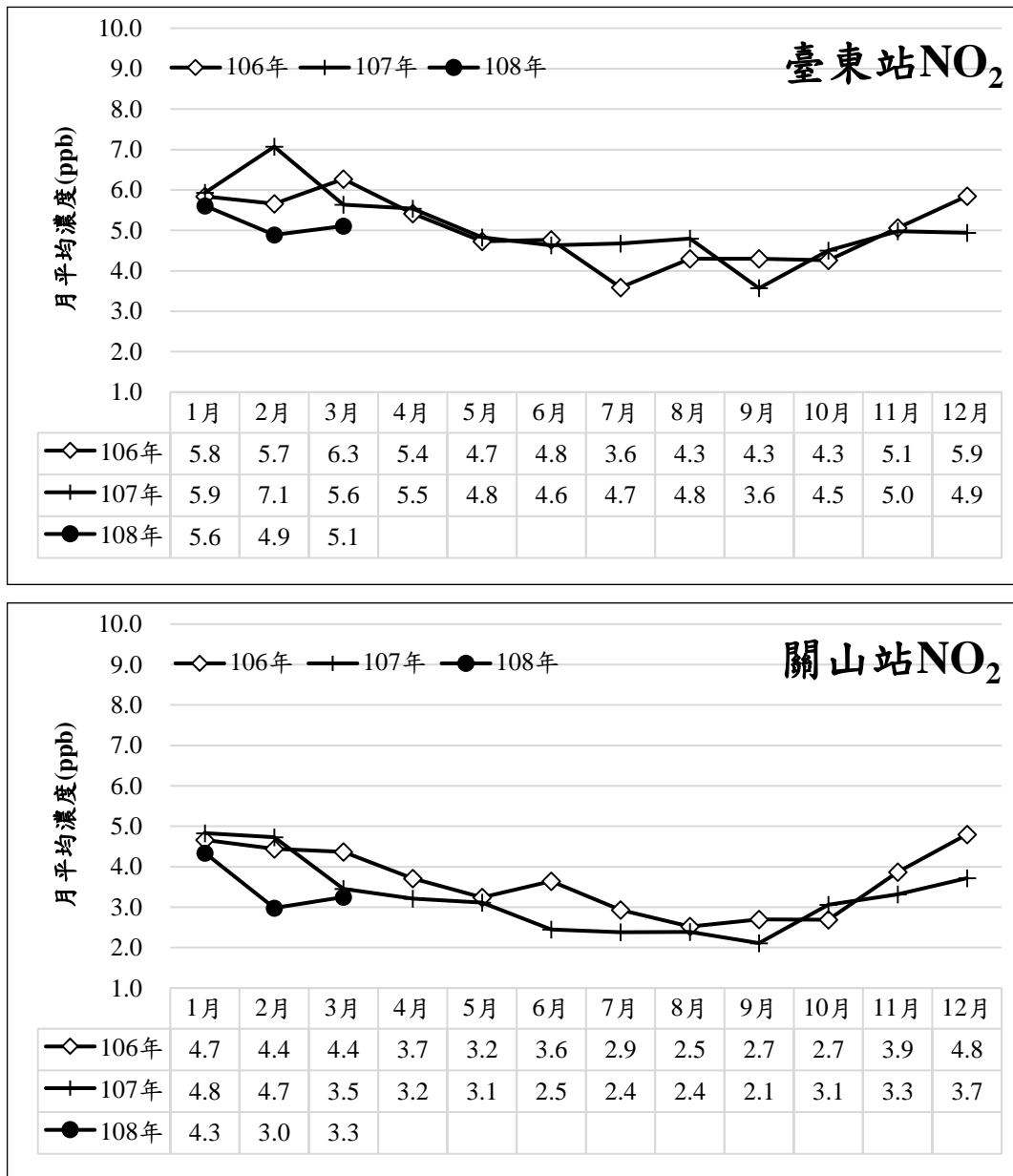
圖 15 近三年 NO 2 濃度逐月變化趨勢
