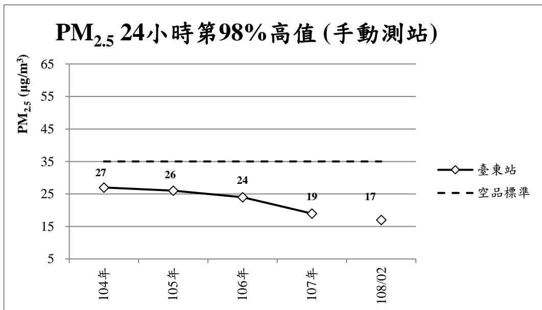
圖 18 臺東環保署測站 PM 2.5 達標程度變化
