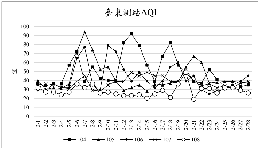
圖 1 近五年 2 月份同期之臺東站空氣品質指標 (AQI) 變化趨勢
