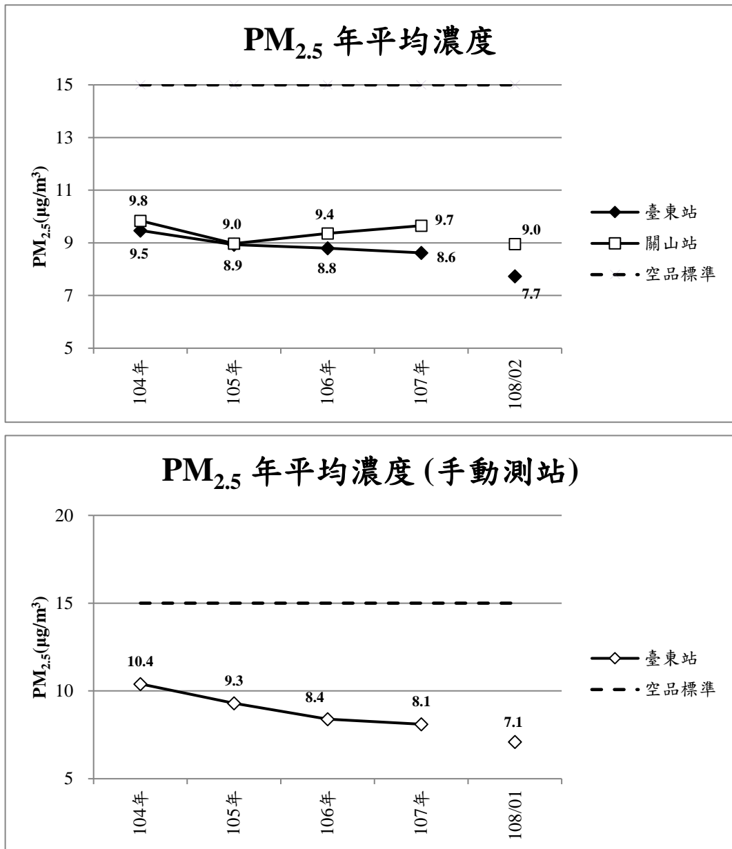
圖 16 臺東環保署測站 PM 2.5 年平均濃度變化
