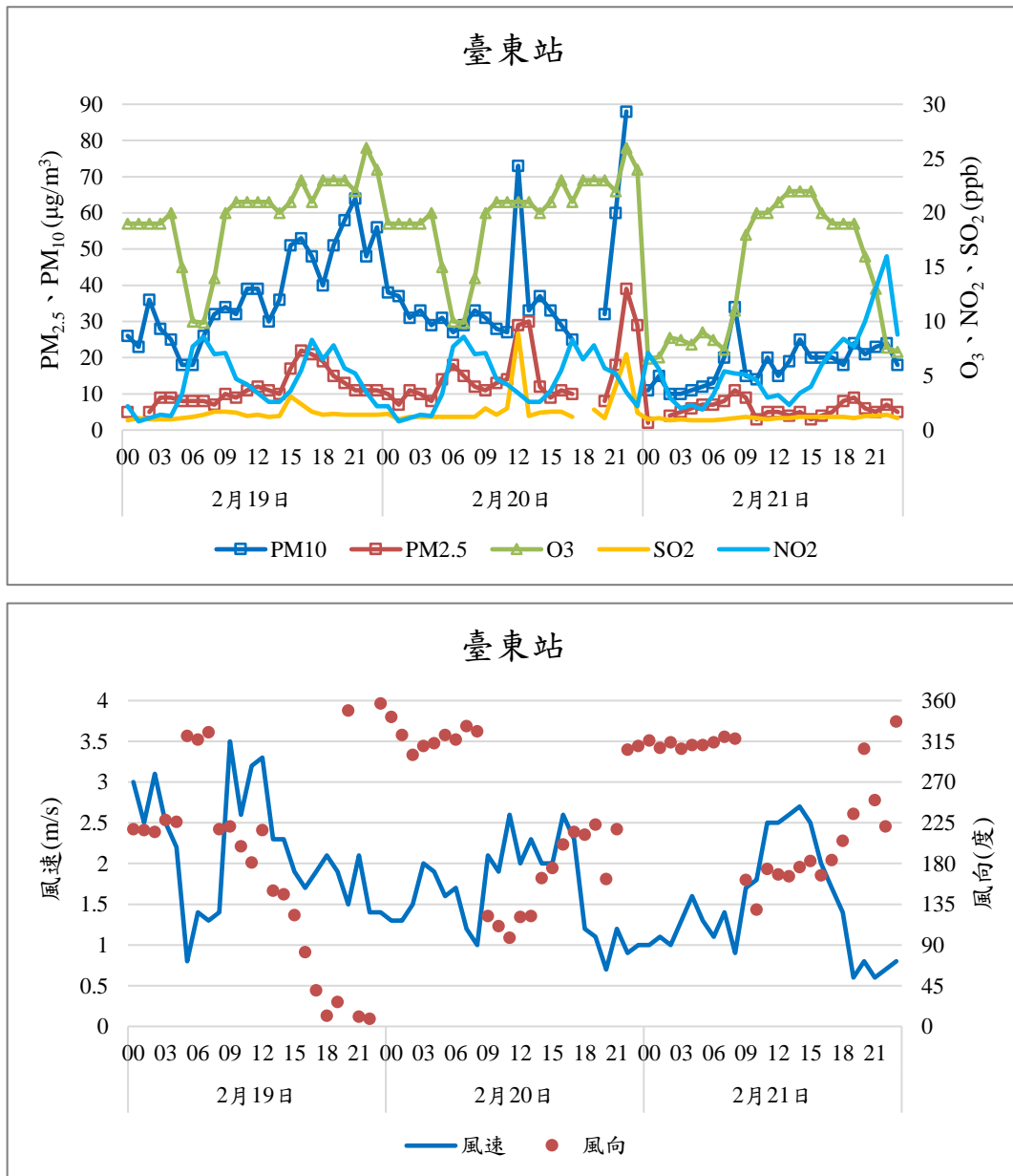
圖 19 2月19~21日臺東站受元宵遶境活動影響之濃度變化情形
