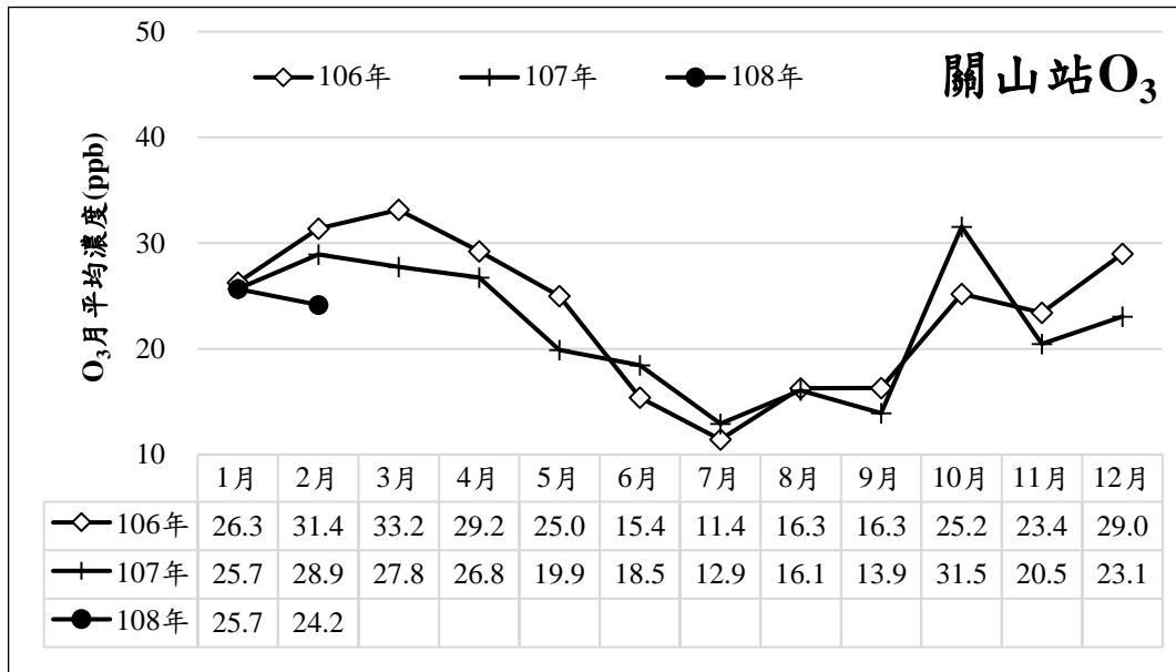
圖 10 近三年 O 3 濃度逐月變化趨勢
