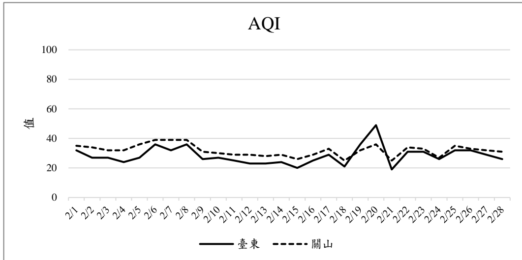
圖 3 108 年 2 月臺東及關山測站空氣品質指標 (AQI) 變化趨勢
