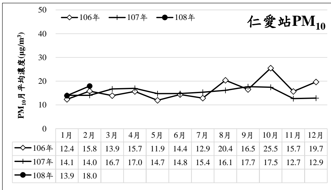
圖 7 近三年 PM 10 濃度逐月變化趨勢
