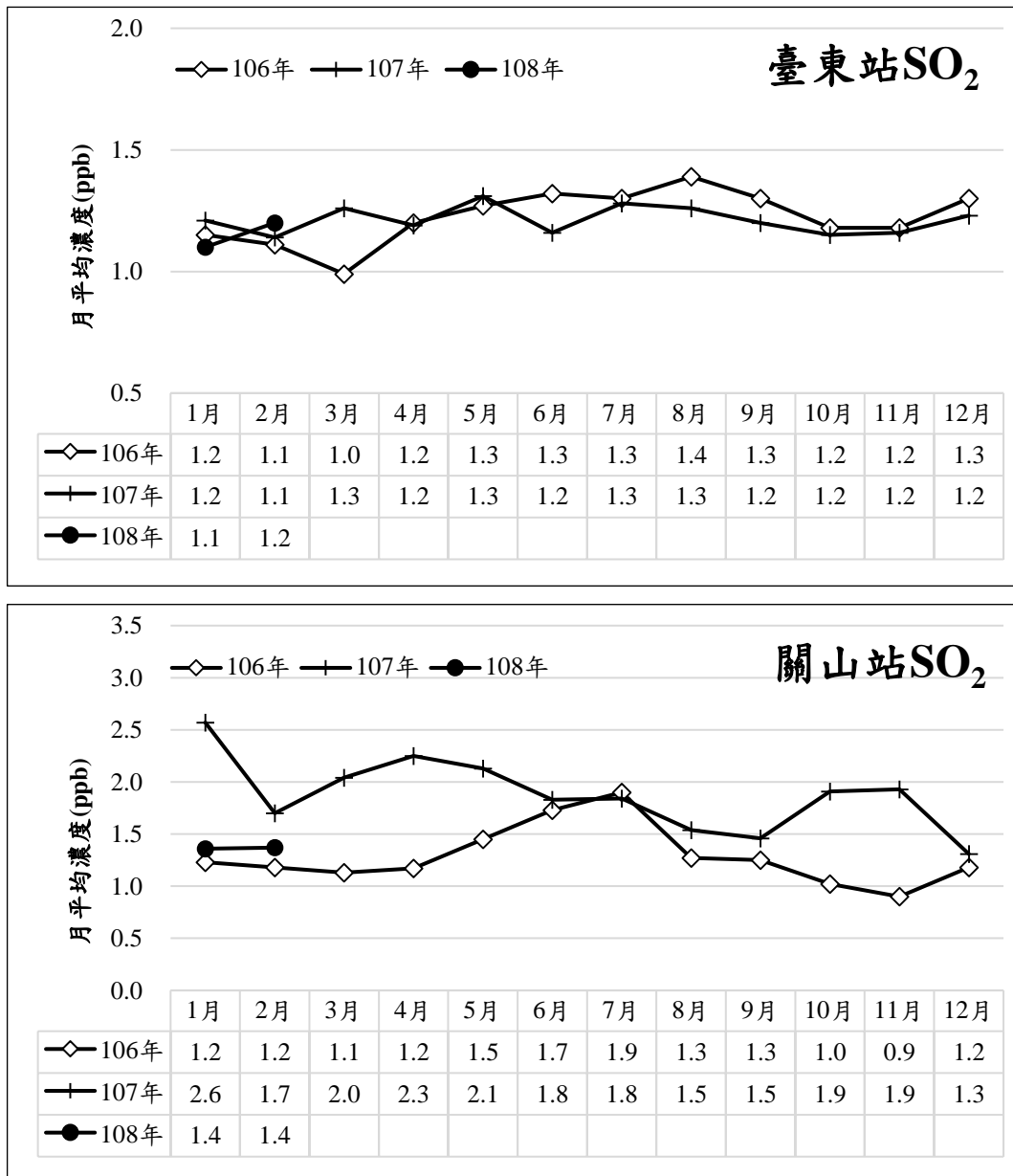
圖 13 近三年 SO 2 濃度逐月變化趨勢
