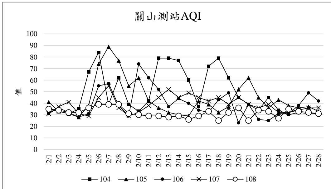
圖 2 近五年 2 月份同期之關山站空氣品質指標 (AQI) 變化趨勢
