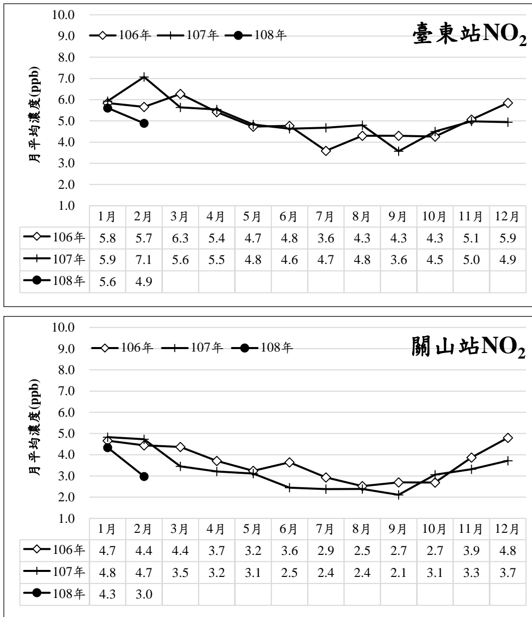
圖 14 近三年 NO 2 濃度逐月變化趨勢
