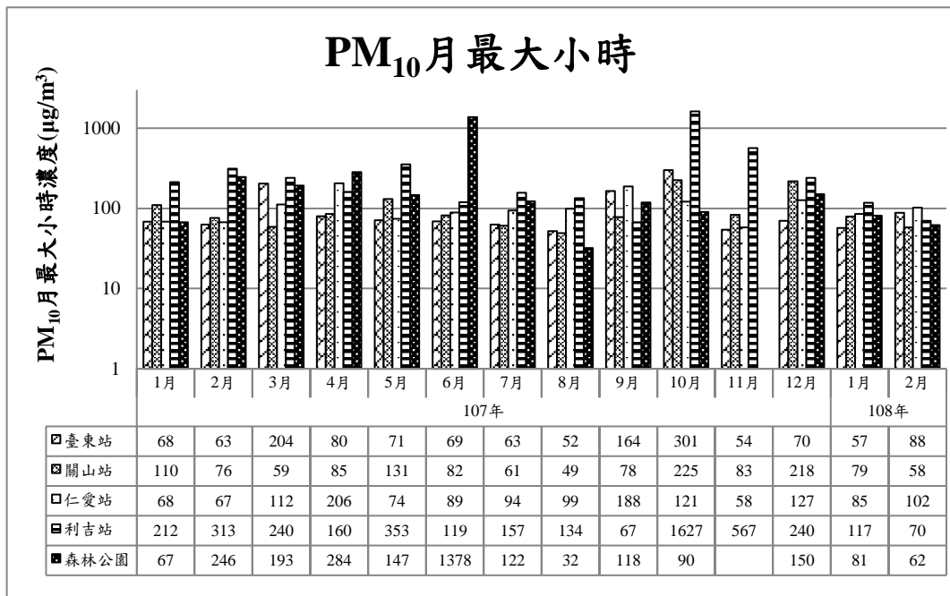
圖 8 各測站 PM 10 濃度月最大小時值變化趨勢
