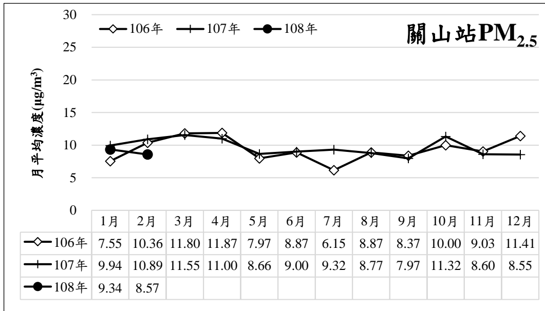
圖 18 近三年 PM 2.5 濃度逐月變化趨勢
