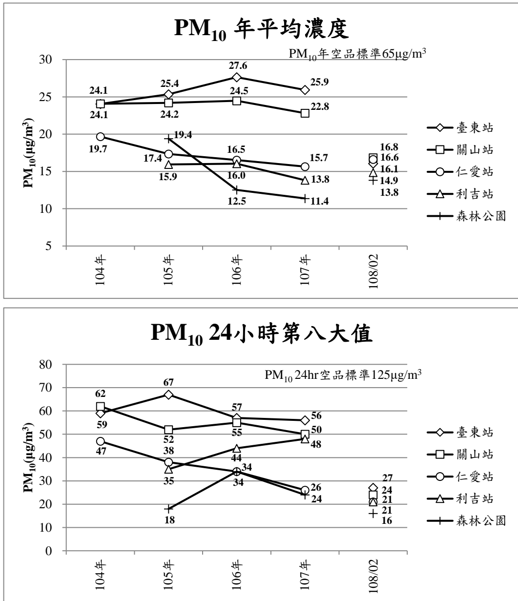
圖 6 臺東環保署測站 PM 10 濃度變化
