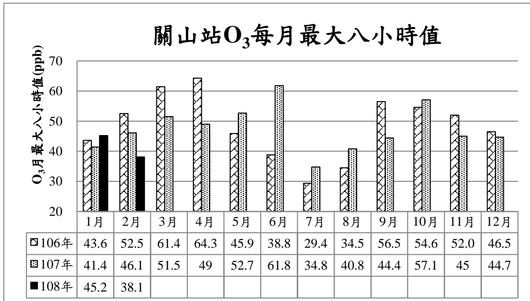
圖 12 近三年 O 3 濃度月最大八小時值變化趨勢
