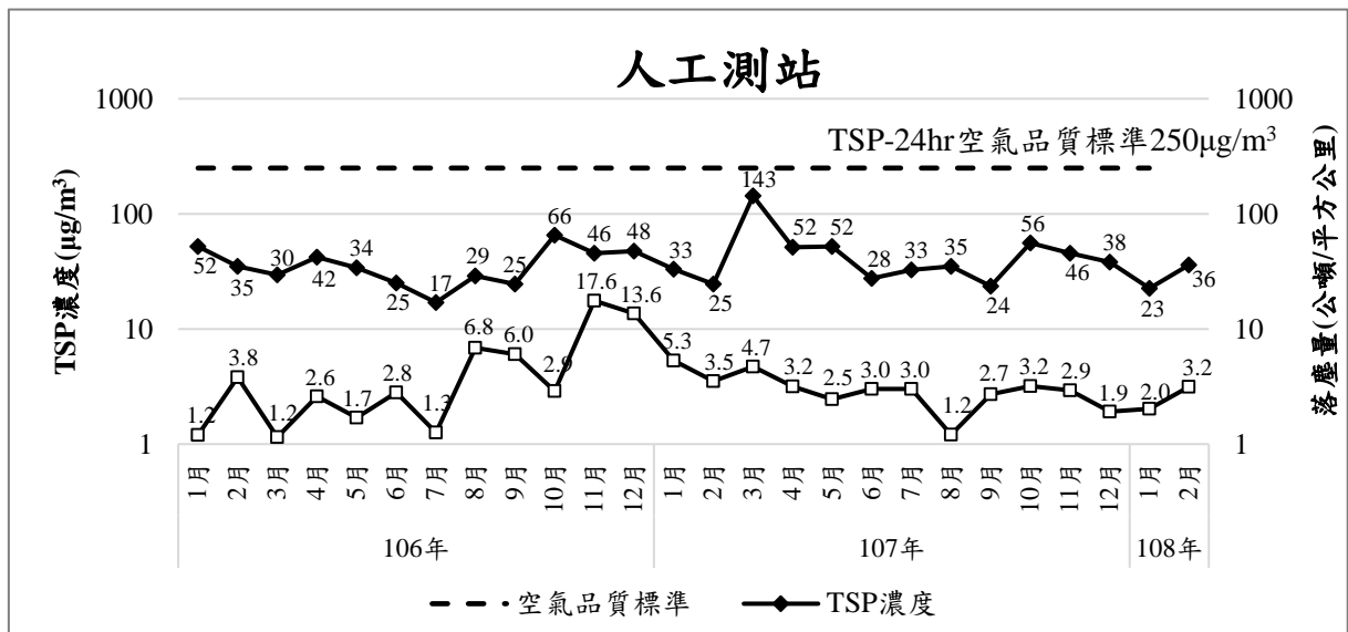
圖 20 臺東環保局人工測站 TSP 與落塵量
