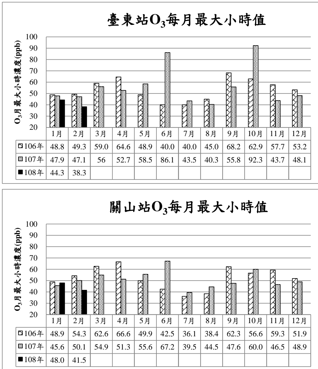
圖 11 近三年 O 3 濃度月最大小時值變化趨勢
