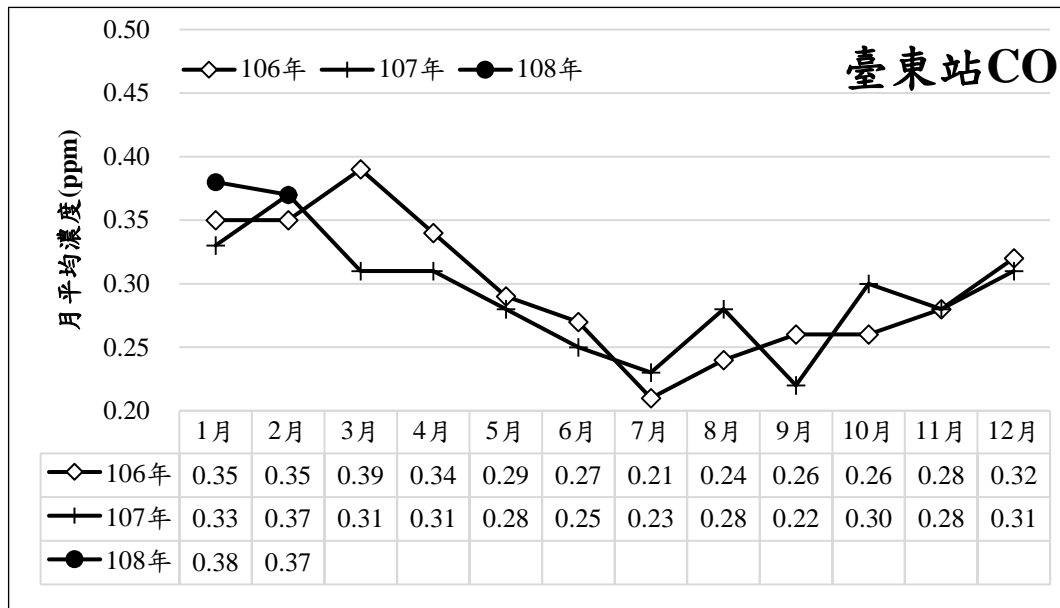
圖 15 近三年 CO 濃度逐月變化趨勢
