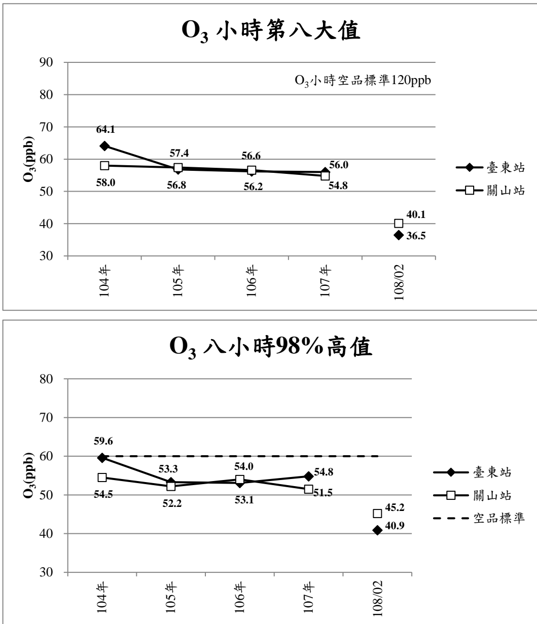
圖 9 臺東環保署測站 O 3 達標程度變化
