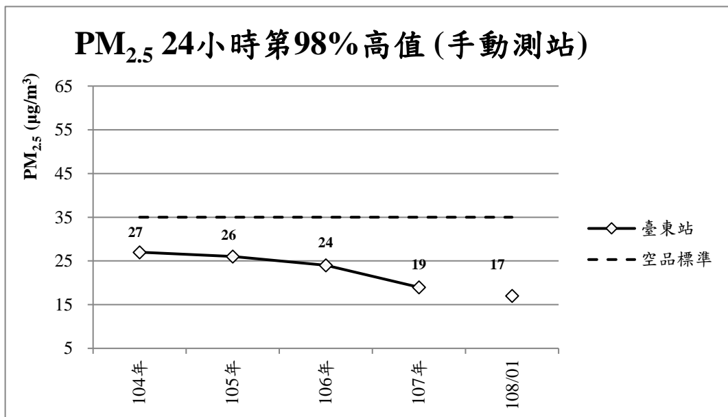
圖 17 臺東環保署測站 PM 2.5 達標程度變化
